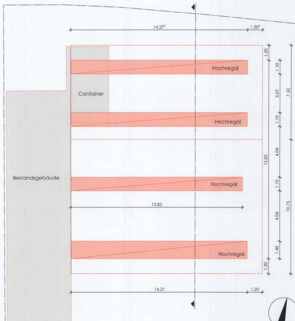
GRUNDRISS
