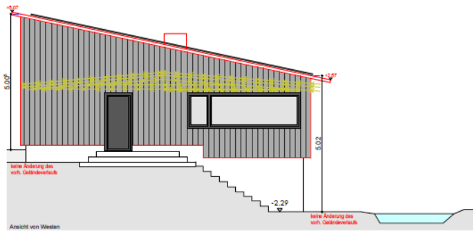
Ansichten 1:100
