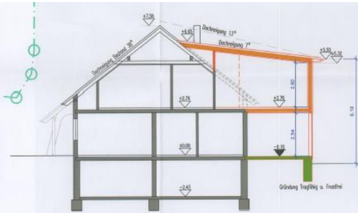
SCHNITT
