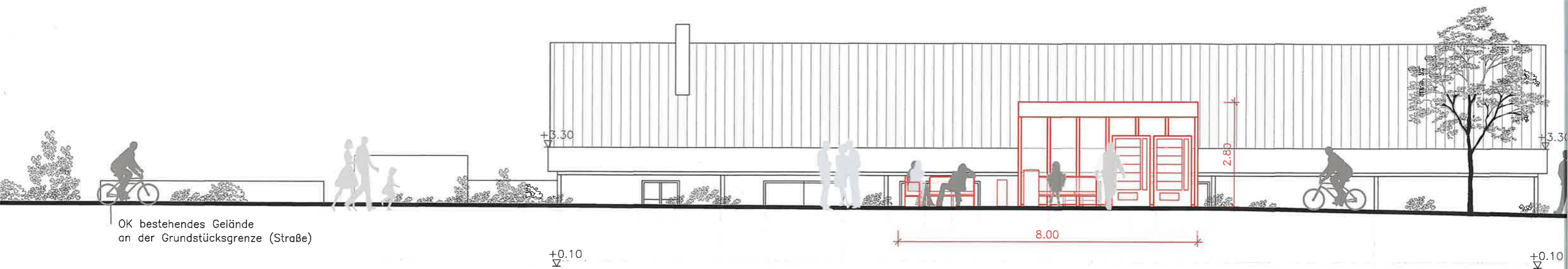
Ansicht Norden
